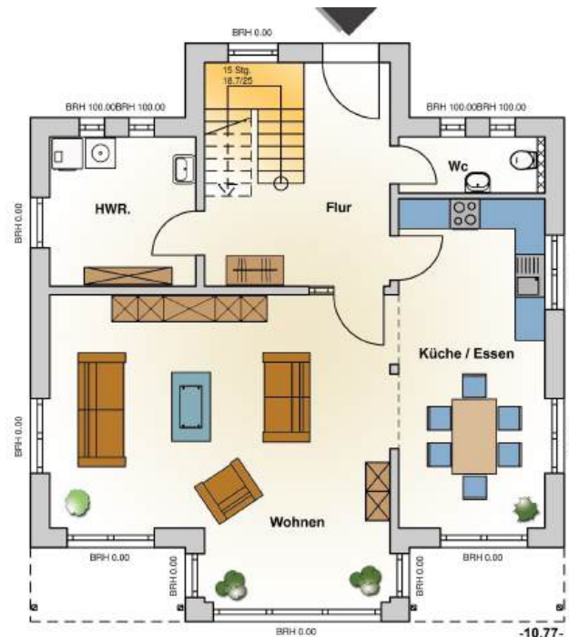
Erdgeschoss
