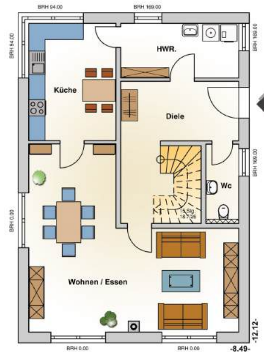
Erdgeschoss
