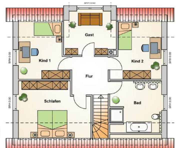
Dachgeschoss
