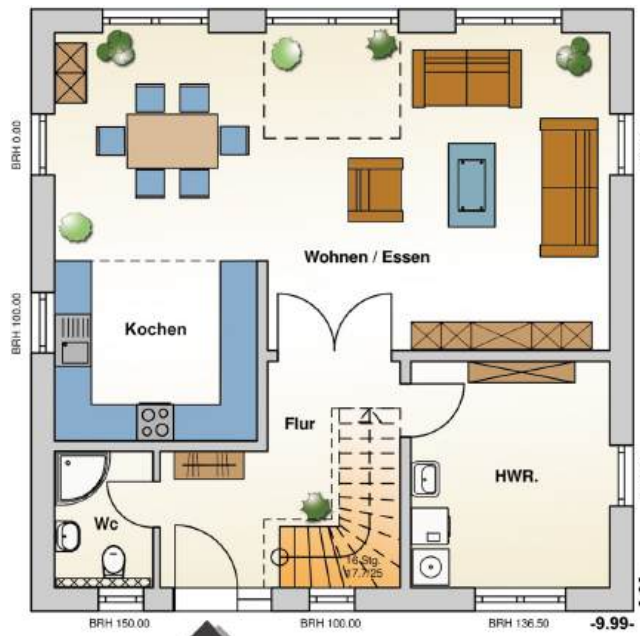
Erdgeschoss
