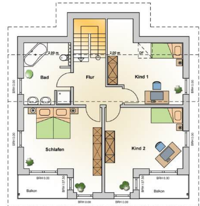
Obergeschoss
