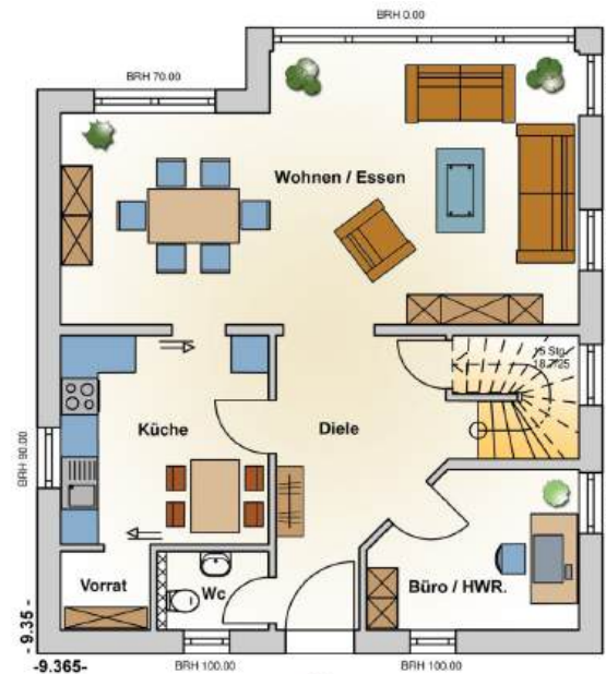
Erdgeschoss
